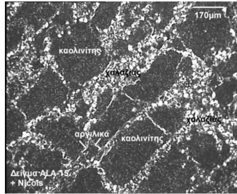
Φωτ. 4: καοлинιτωμένο ηφαιστειοκλαστικό πέτρωμα, (πολωτικό μικροσκόπιο, ⊥ Nicols)
