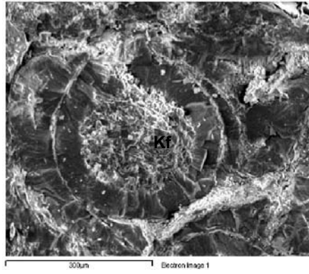
Φωτ. 2: Φωτογραφία SEM, αμιδική κρυστάλλωση Κούχου αστρίου (Kf), σε πόρους γυαλιού με περιλιτική υφή.
