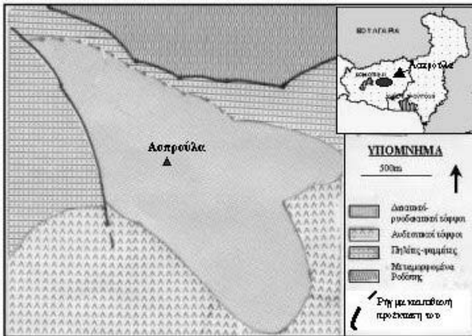
Σχήμα 1. Θέση, γεωλογικός χάρτης περιοχής Ασπρούλα, Ν. Ροδόπης
