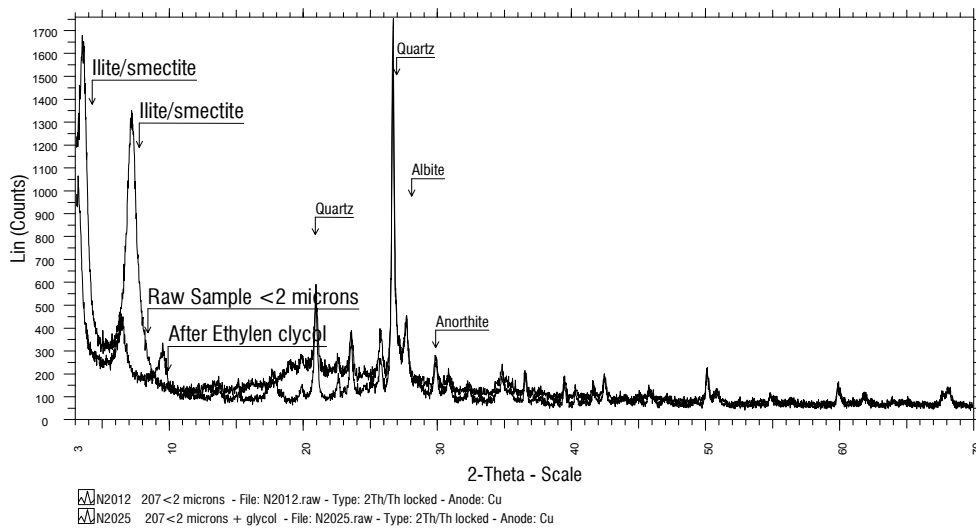
Σχήμα 3: Διάγραμμα περιθλασιμετρίας ακτίνων Χ, κλάσματος <2μ τόφφων εξαλλοιωμένων σε αργίλικά μικτών δομικών μονάδων ιλλίτη-σμεκτίτη. (κλάσμα 2μ φυσικό, μετά από κατεργασία με αιθυλενογλυκόλη).
